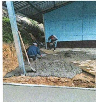
Foto 2: Mejoramiento de torta de cemento para que los niños y niñas tengan una superficie de piso evitando la tierra y el polvo.
